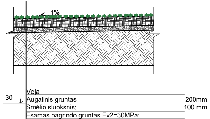
Detalė Nr. 2 Pjūvis B-B Sporto aikštelė su vejos danga
