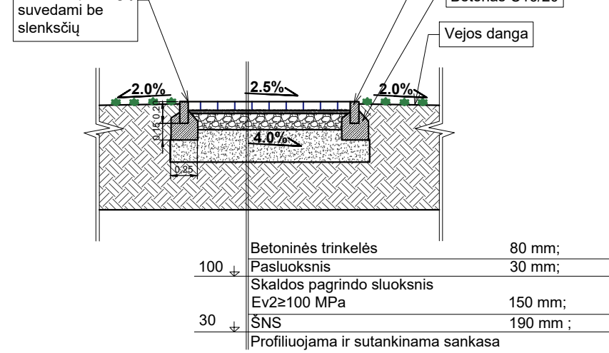
Detalė Nr. 5 Pjūvis E-E Pėsčiųjų plytelių danga
