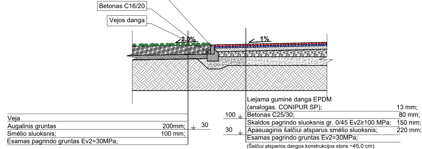
Detalė Nr. 4 Pjūvis D-D Sporto aikštelė su betono pagrindu ir 2 sl. liejama gumos granuliu ir vejos danga
