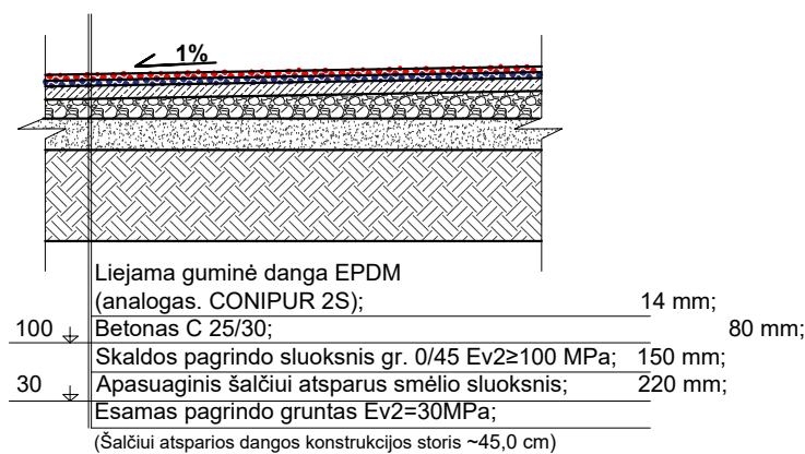
Detalė Nr. 1 Pjūvis A-A (aikštelės) Sporto aikštelė su betono pagrindu ir 2 sl. liejama gumos granuliu danga
