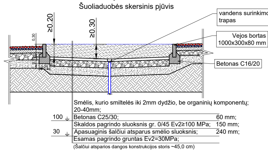
Detalė Nr. 6 Pjūvis F-F Šuoliadubės skersinis pjūvis
