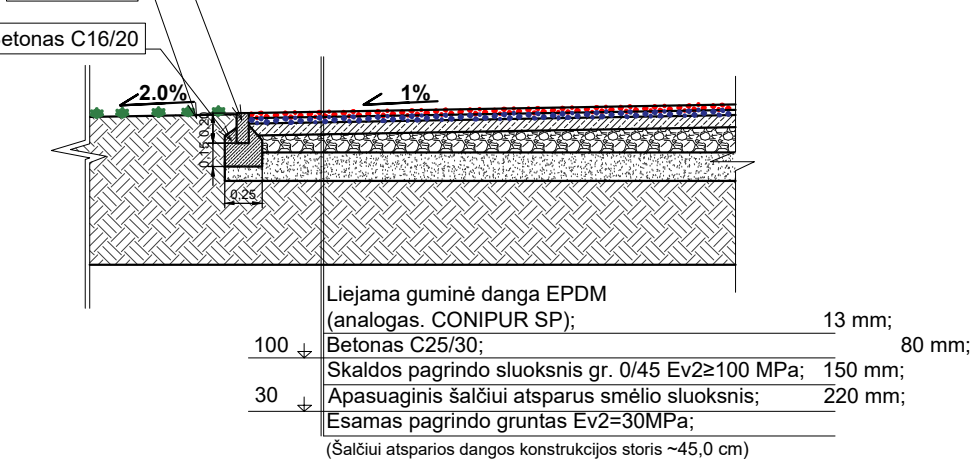
Detalė Nr. 3 Pjūvis C-C (bėgimo takai) Sporto aikštelė su betono pagrindu ir 2 sl. liejama gumos granuliu danga
