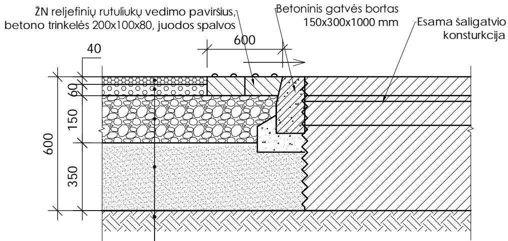
PJŪVIS 4-4 M 1:20
