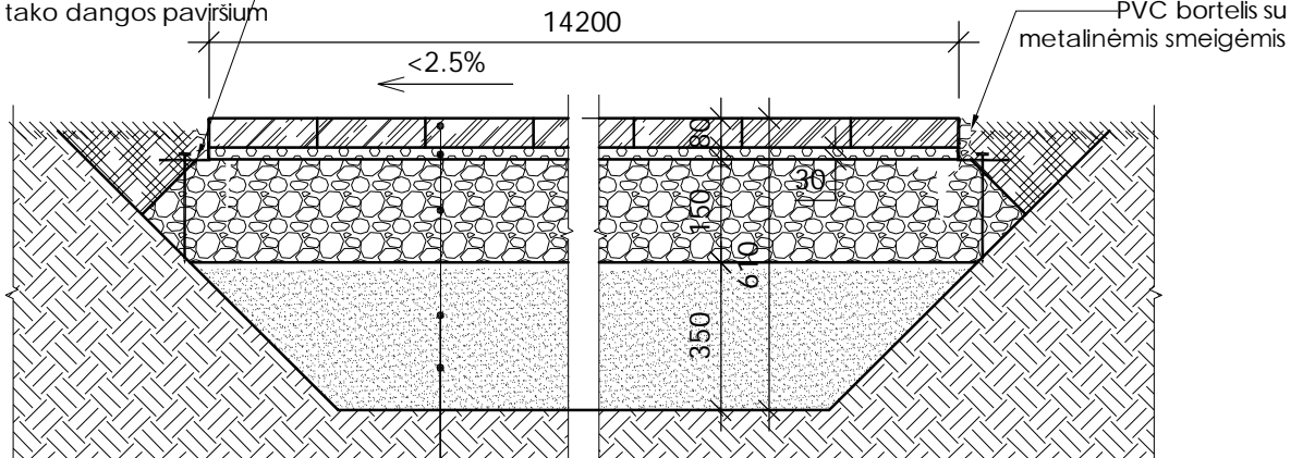
PJŪVIS 2-2 M 1:20
