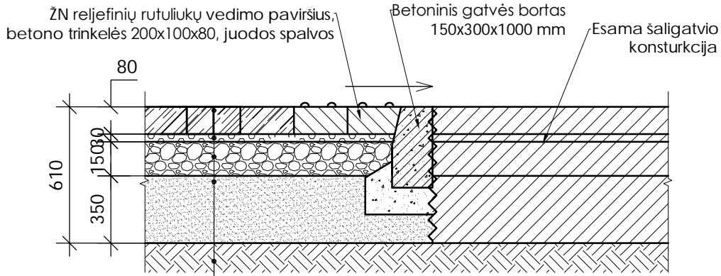
PJŪVIS 3-3 M 1:20
