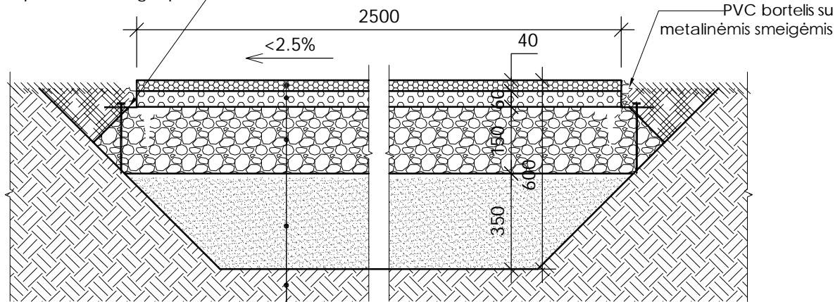
PJŪVIS 1-1 M 1:20
